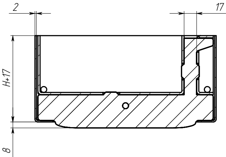
СЕЧЕНИЕ D-D (1 : 3)
